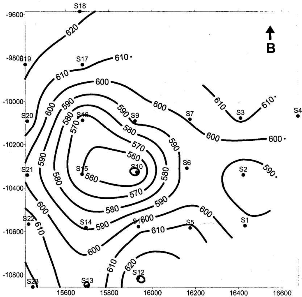
Σχ. 3: Χάρτης στον οποίο φαίνεται το ανάγλυφο του αλπικού υποβάθρου, της πόλης της Πόλιανης.
