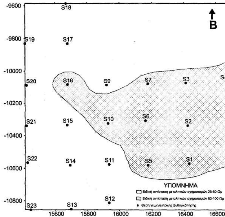
Σχ. 6: Χάρτης γεωγραφικής κατανομής του ενδιάμεσου στρώματος των μεταλλικών σχηματισμών της πόλης. (α) ειδική αντίσταση 25-60 Ω·m, που αντιστοιχεί είτε στην παρουσία λεπτόκοκκων υλικών, είτε στην ανάπτυξη υδροφορίας και (β) ειδικής αντίστασης 60-100Ω·m, που αντιστοιχεί σε αδρομερή σχηματισμό χωρίς υδροφορία.
