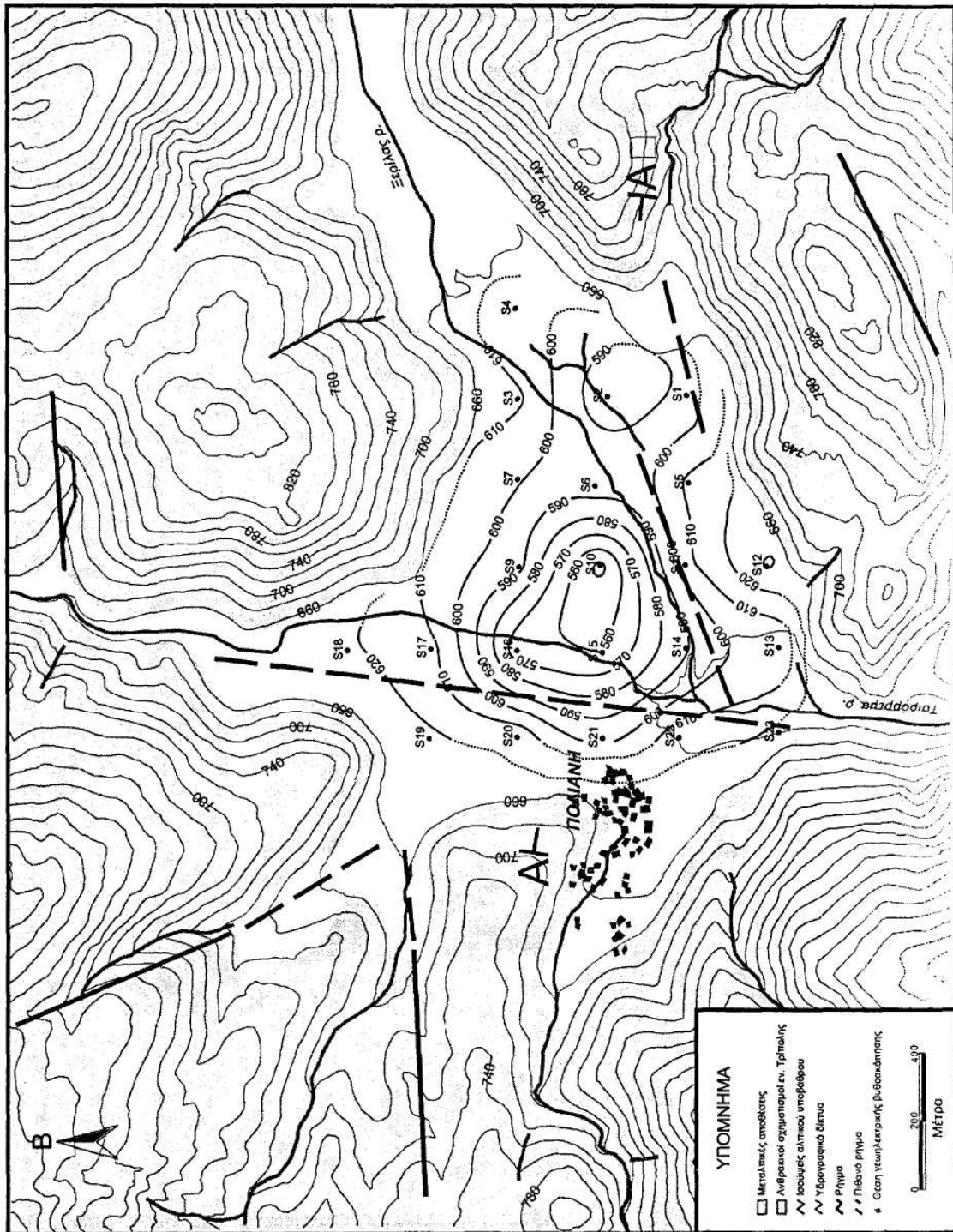
Σχ. 2: Τοπογραφικός χάρτης της πόλης της Πολιανής και μορφολογικός χάρτης του αλικού υποβάθρου, με τις οι θέσεις των γεωηλεκτρικών βυθοσκοπήσεων.
