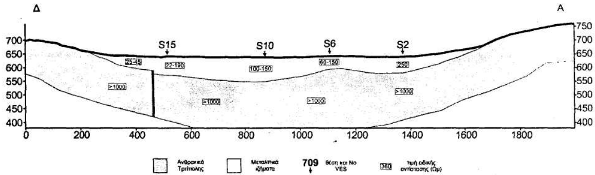
Σχ. 5: Γεωλογική-γεωφυσική τομή ΑΑ'.
