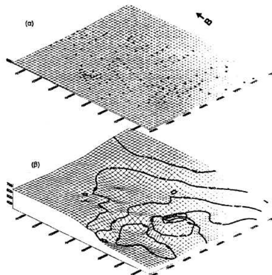
Σχ. 7: Τρισδιάστατη απεικόνιση αναγλύφου του μορφολογικού (α) και αλπικού υποβάθρου (β), της λεκάνης της Τρίπολης, σε κλίμακα 1:1:3.
