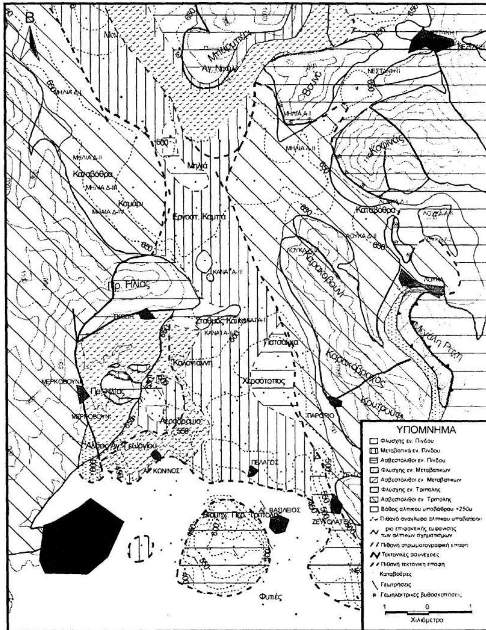
Σχ. 2: Γεωλογικός χάρτης επιφανειακών και υπεδαφικών εμφανίσεων των γεωλογικών σχηματισμών.
