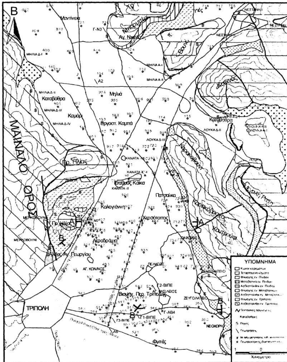
Σχ. 1: Γεωλογικός χάρτης της περιοχής μελέτης στον οποίο απεικονίζονται οι θέσεις των επιτόπιων μετρήσεων και των γεωηλεκτρικών βυθοσκοπήσεων.
