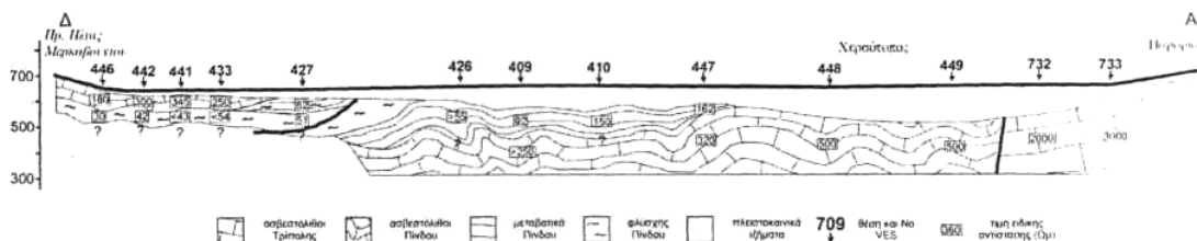
Σχ. 4: Γεωλογική τομή ΑΑ', στην κεντρική περιοχή της λεκάνης της Τρίπολης, όπως προέκυψε μετά την εκτέλεση των γεωηλεκτρικών βυθοσκοπήσεων.
